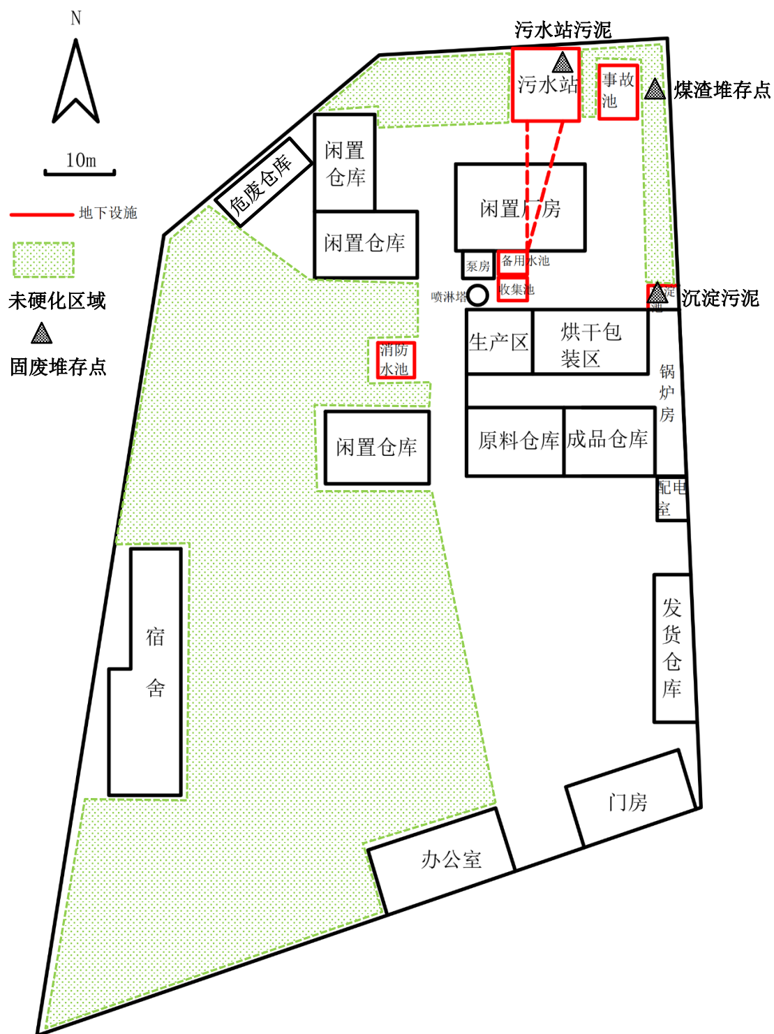
图 3.3-2 项目平面布置图
