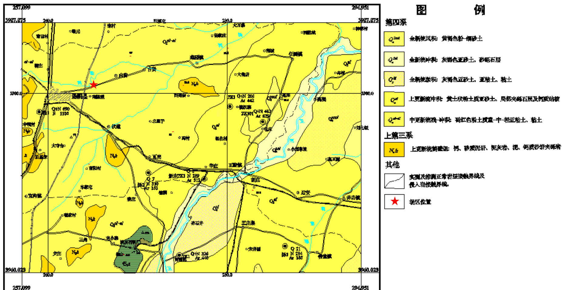
图3.1-4 区域地层结构图
