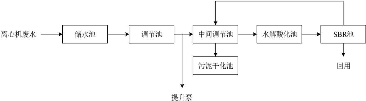
图 3.3-4 项目污水处理工艺流程图
