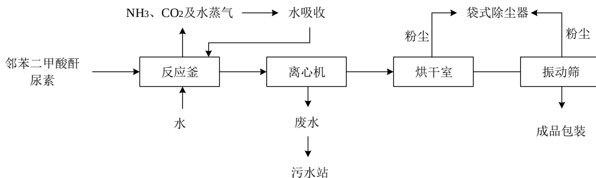
图 3.3-3 企业生产工艺流程图
