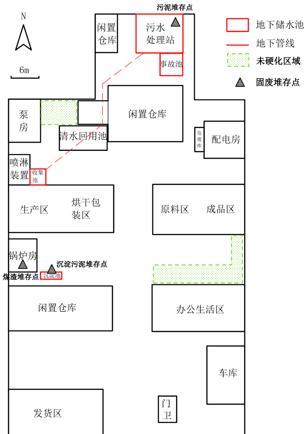
图 3.3-3 项目平面布置图
