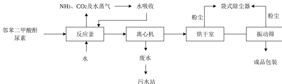
图 3.3-4 企业生产工艺流程图
