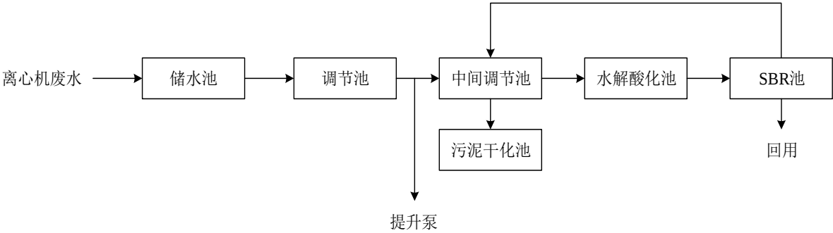
图 3.3-5 项目污水处理工艺流程图
